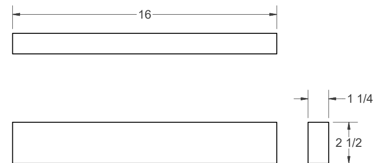
(D) - CLEAT
