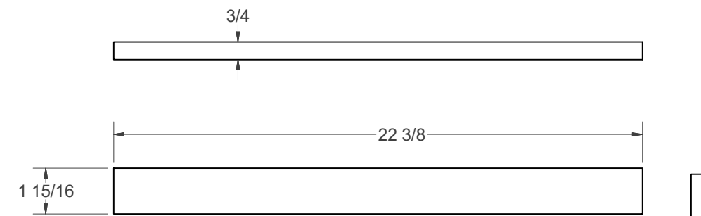
(N) - DIVIDER (2)
