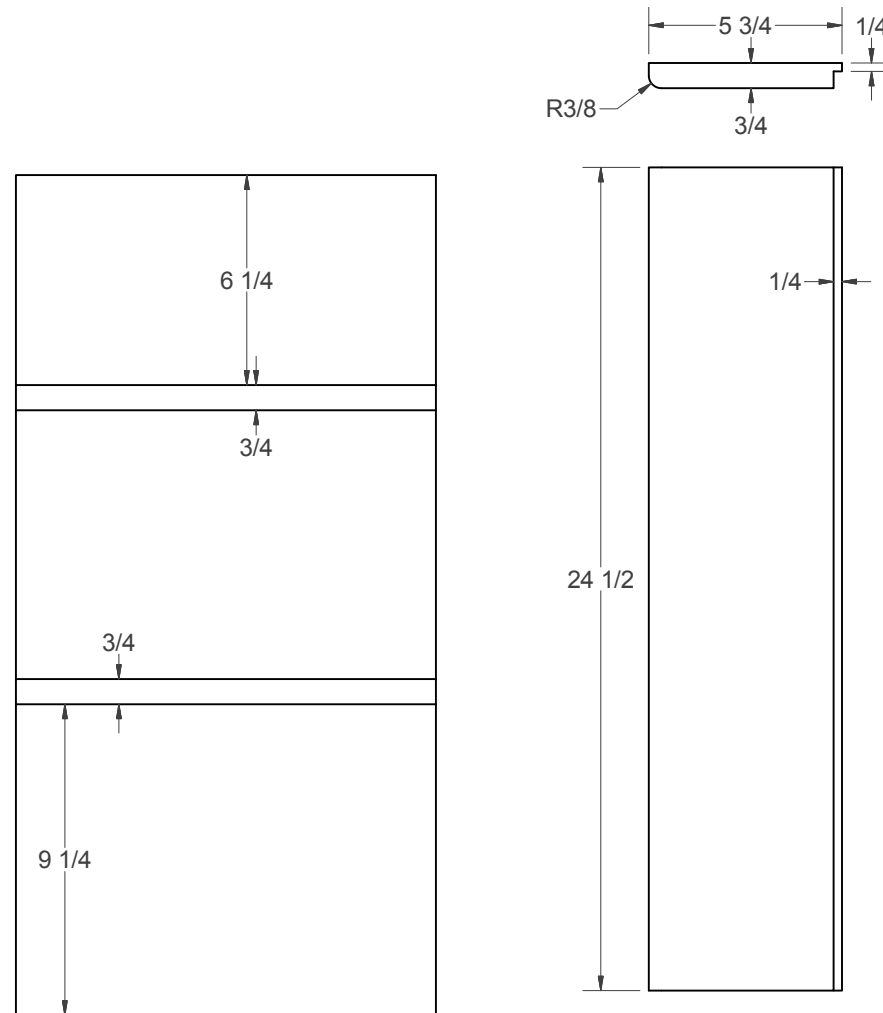
(D) - SIDES (2 PCS)
