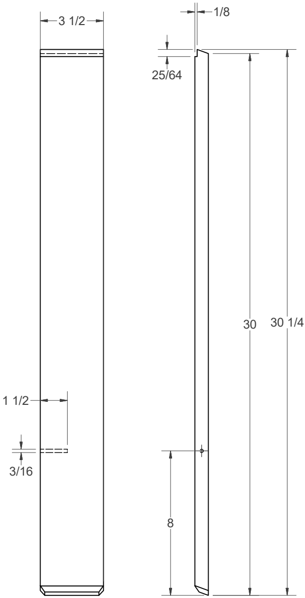
(B) - LEG INSIDE LAYER (4)
