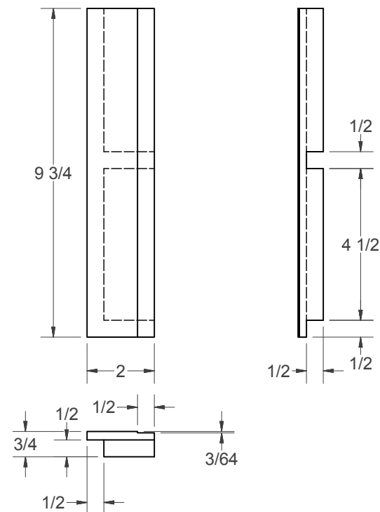
(E) - INNER STILE (x2)
