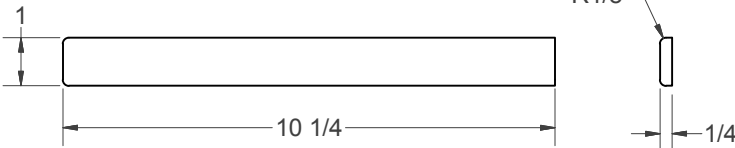
(O) - EDGING (x2)
