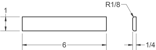
(O) - EDGING (x2)
