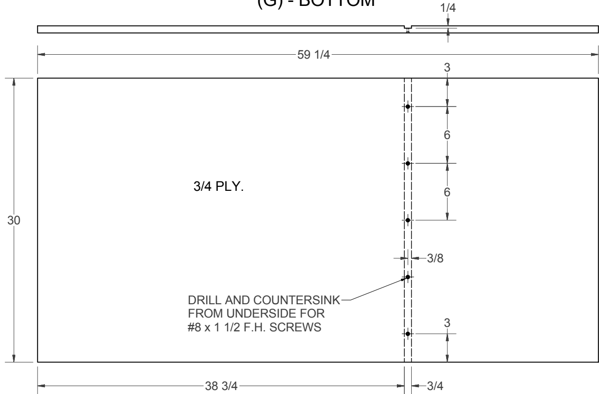
(G) - BOTTOM
