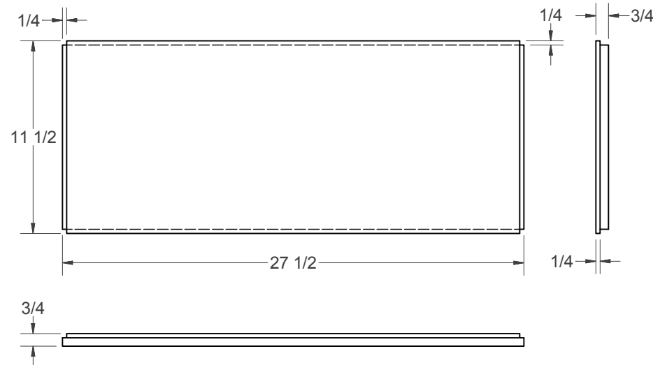
(T) - TOTE BOTTOM (3)
