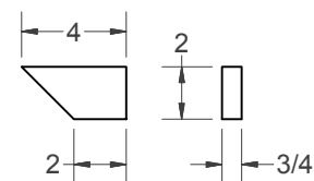
(AA) - BRACE (2)
