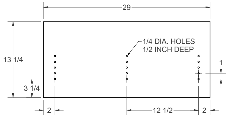
(J) - DIVIDER
