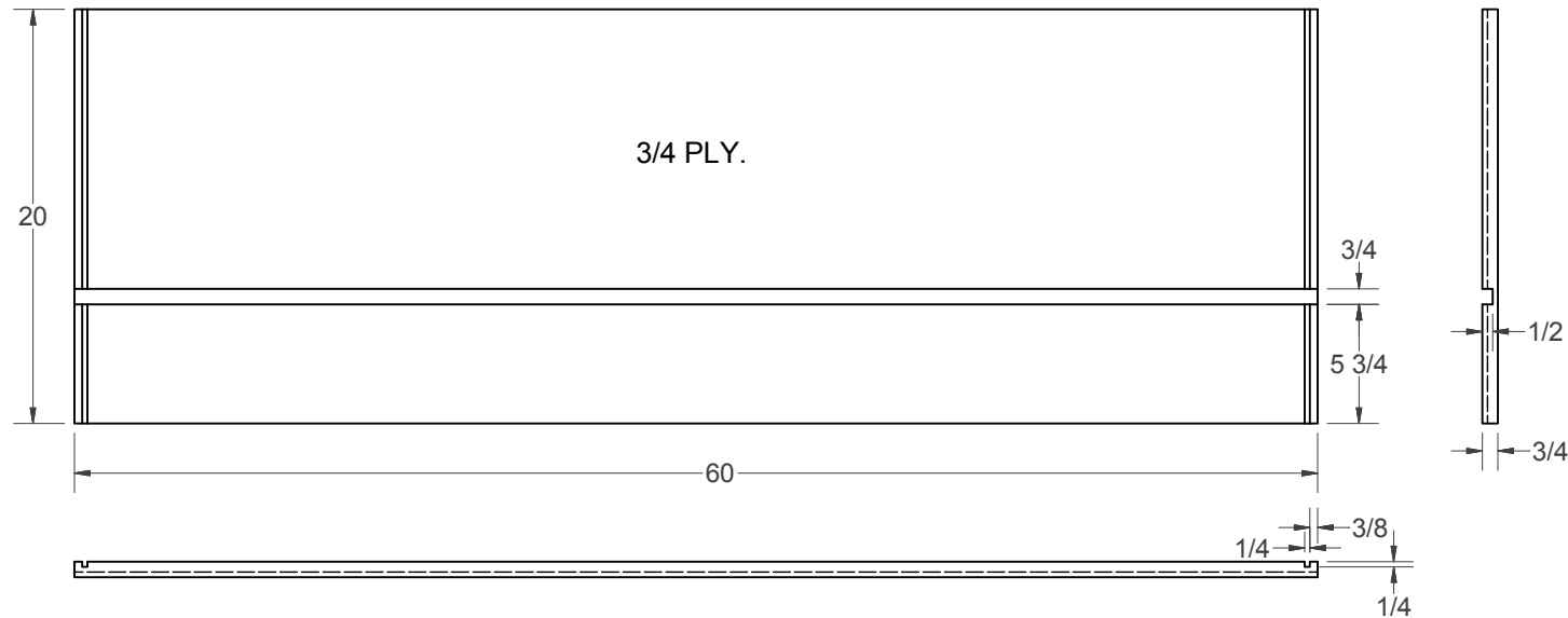
(G) - BOTTOM
