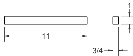
(U) - TOTE CLEAT (6)
