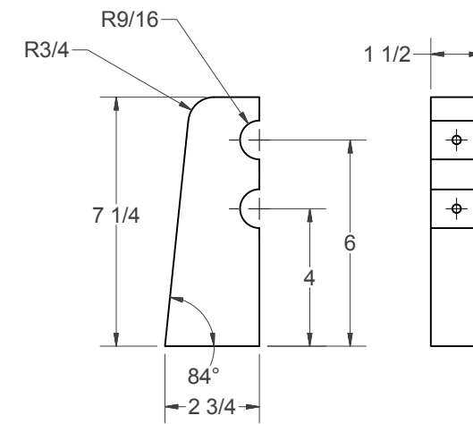
(D) - RISER (4 NEEDED)
