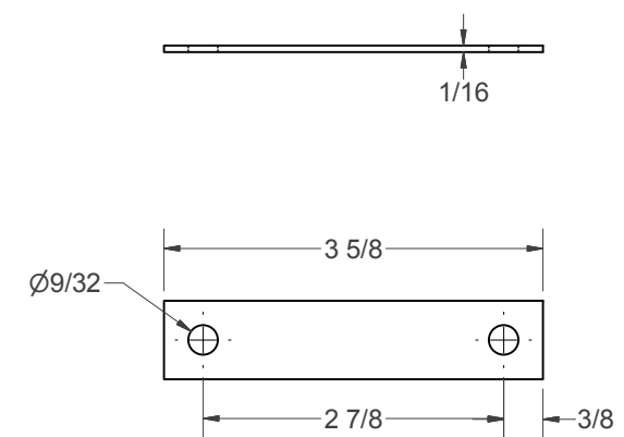
ALUMINUN STRAP SCALE 1 : 1
