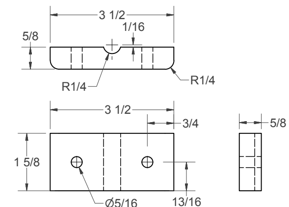
(O) - STYLUS CLAMP
