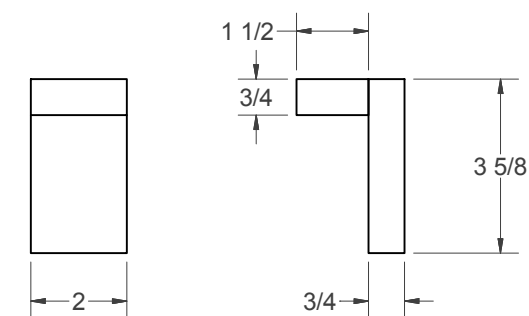
(D) - STOP BASE
