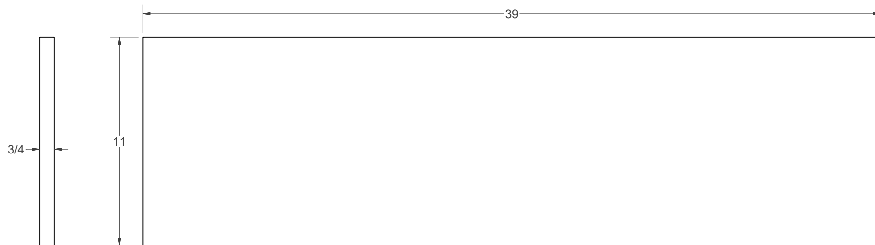
DIVIDER (1)
