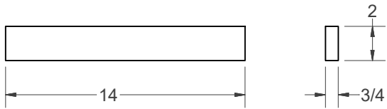
(H) - GUIDE CLEAT
