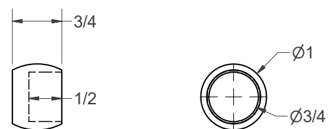
(F) - CAP
