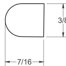
(AA) - DOOR BEAD
