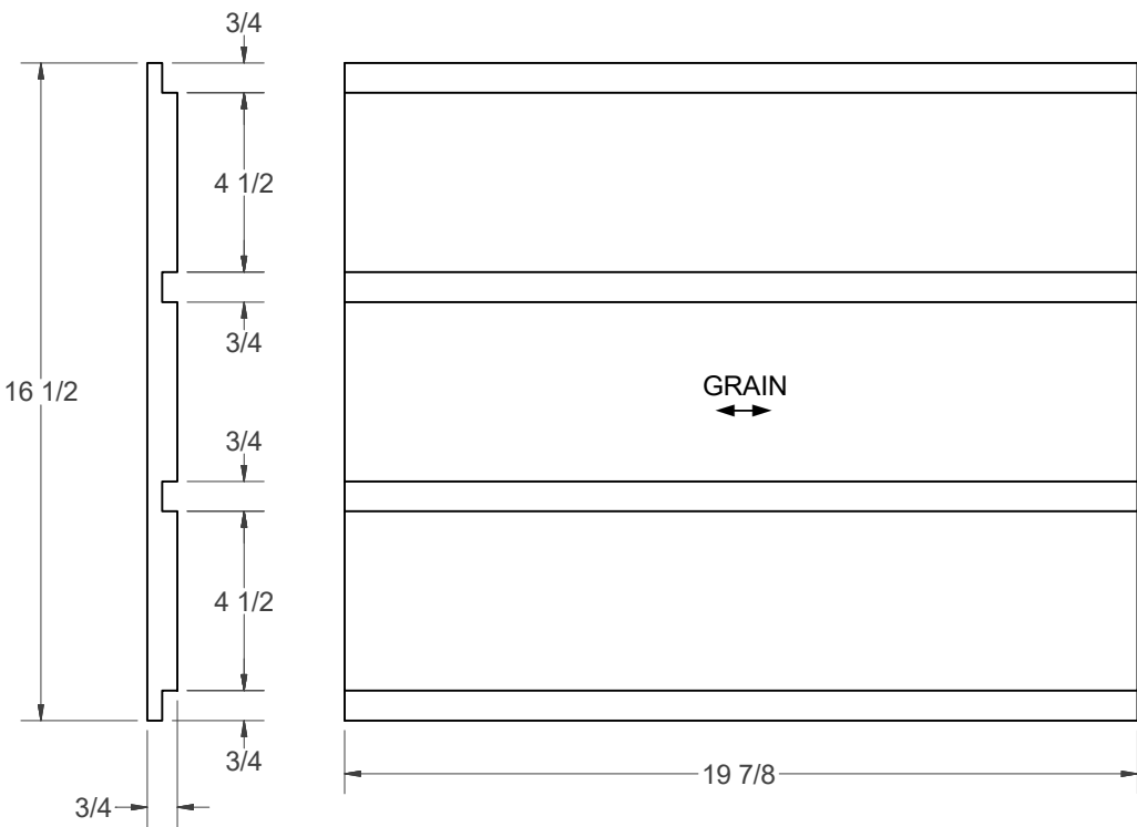
(O) - CASE SIDE (2)
