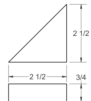
(D) - BRACE (QTY. 4)
