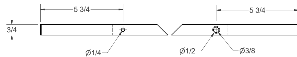
(D) - FENCE
