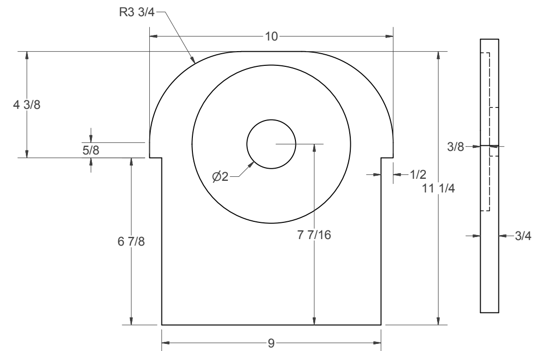
(JJ) - ROUTER BASE
