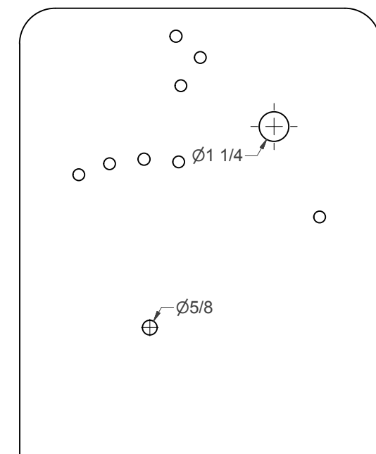
(D) - LEFT SIDE
