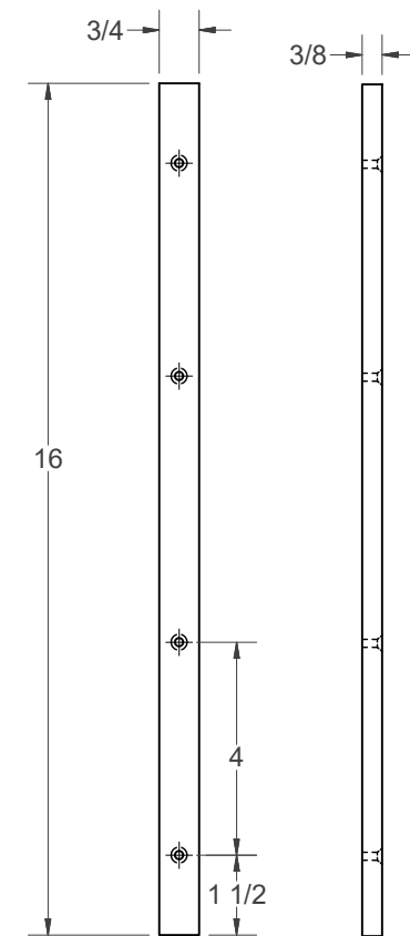
(D) - RUNNER
