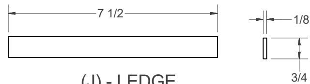
(J) - LEDGE
