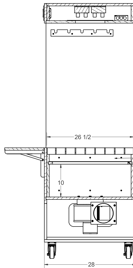
SECTION E-E SCALE 0.14 : 1
