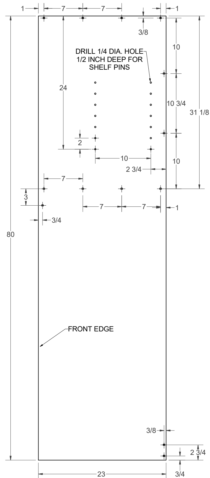
CENTER CAB. LEFT SIDE
