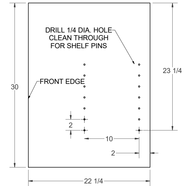
CENTER CAB. DIVIDER
