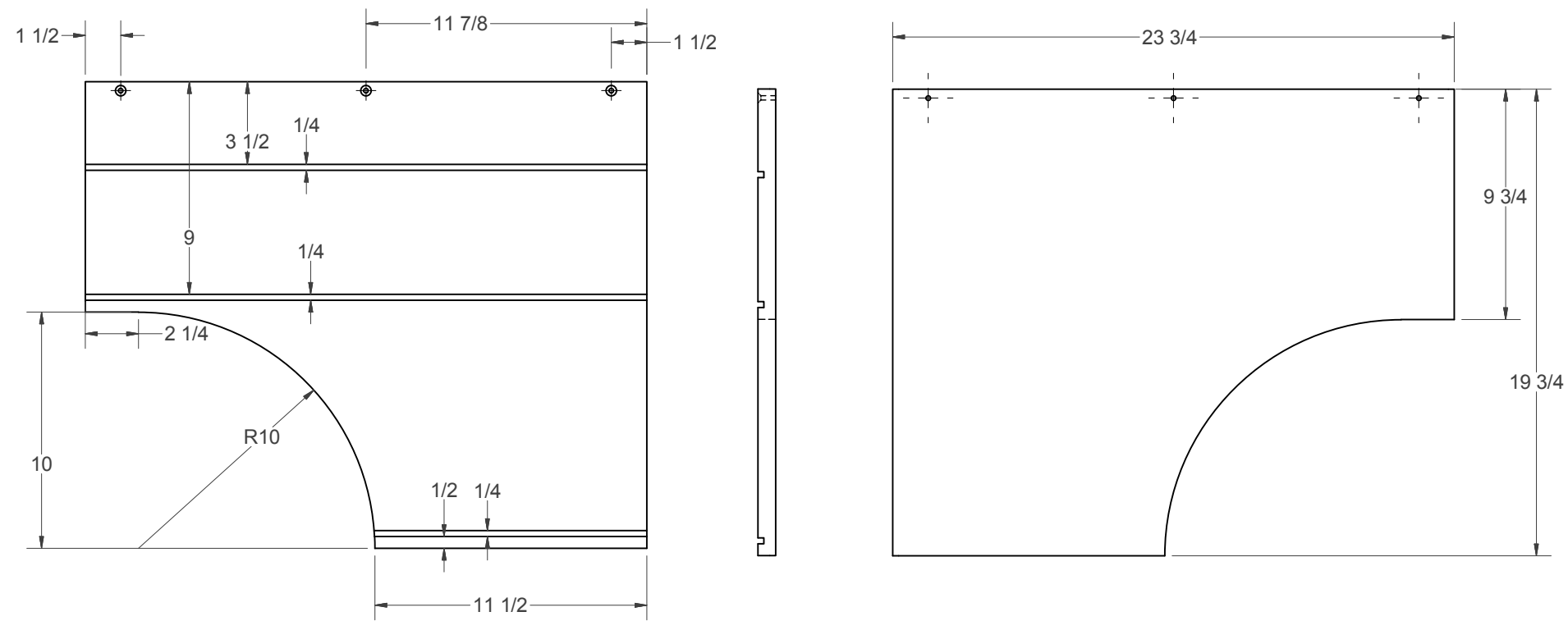
(F) - LEFT SIDE
