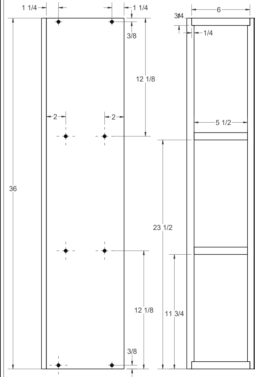
LEFT SIDE
