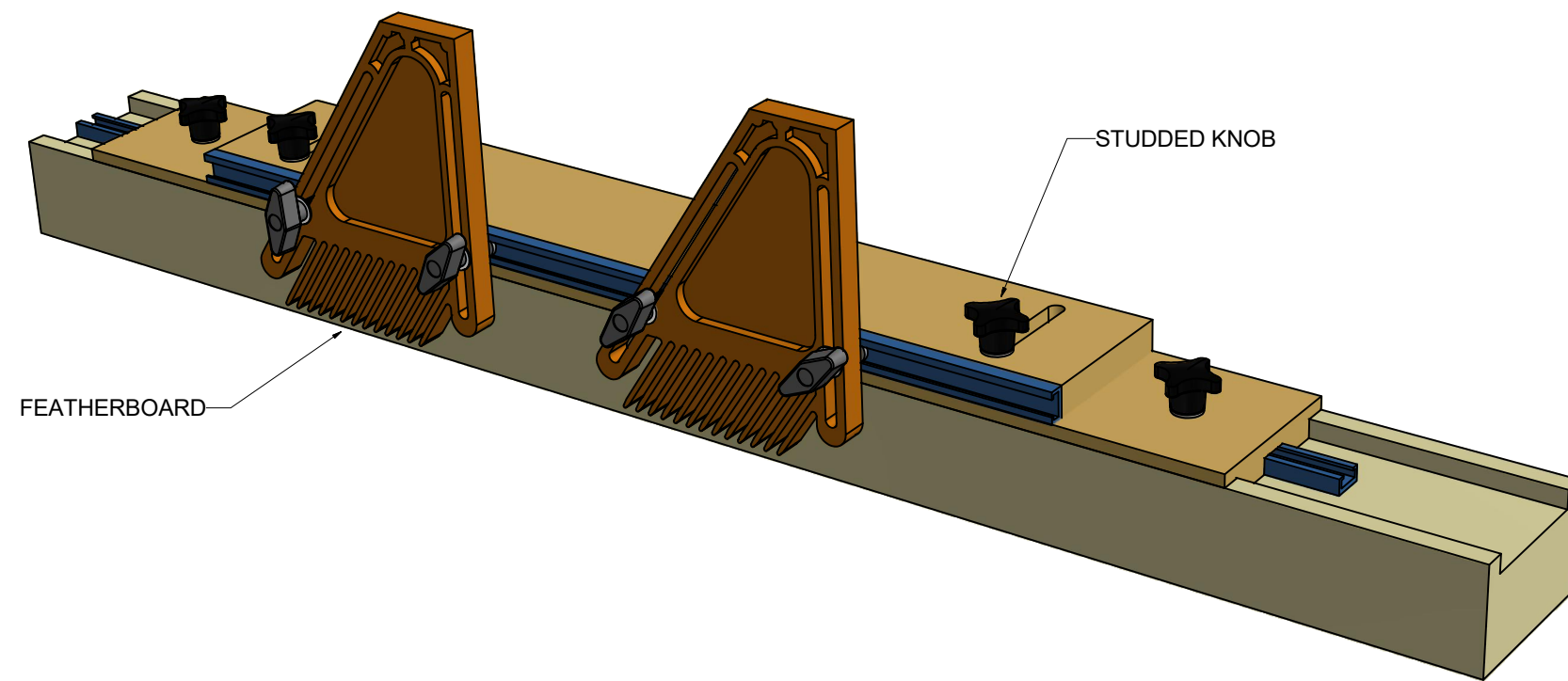
DADO FENCE
