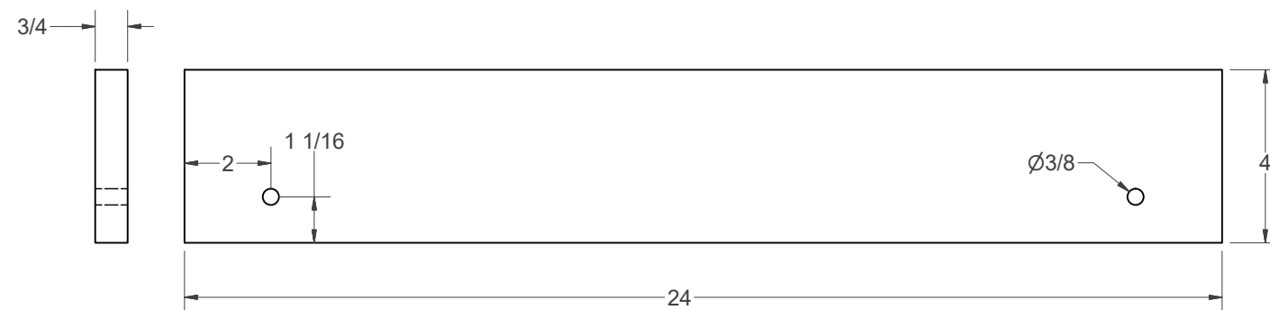
DADO FENCE
