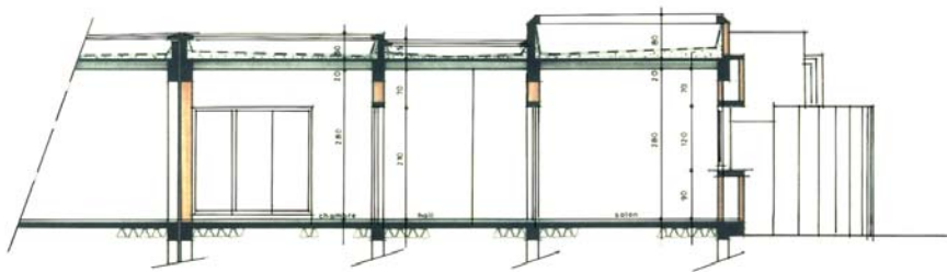
COUPE AA
