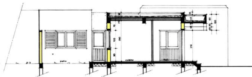
COUPE CC
