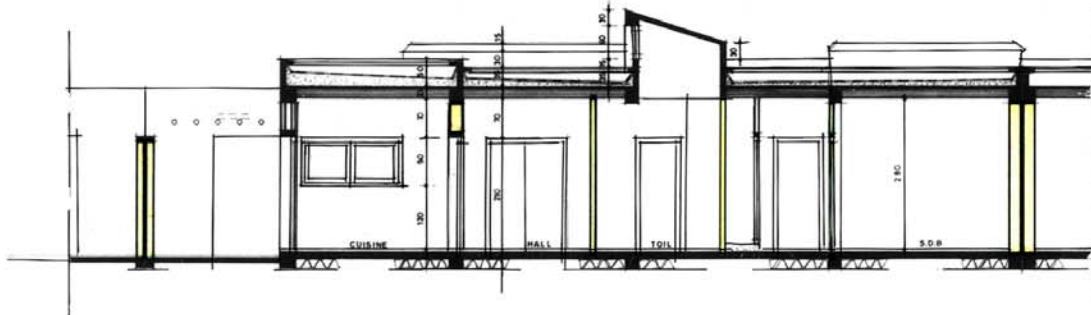
COUPE BB
