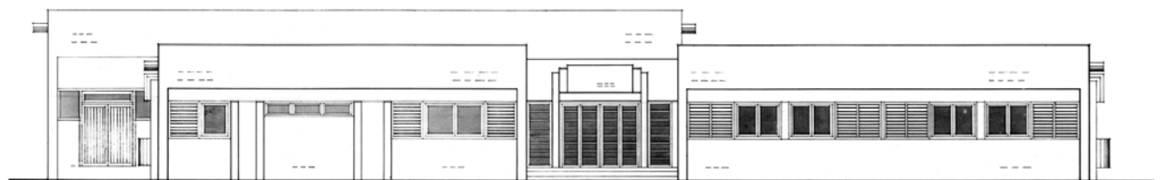
FACADE PRINCIPALE
