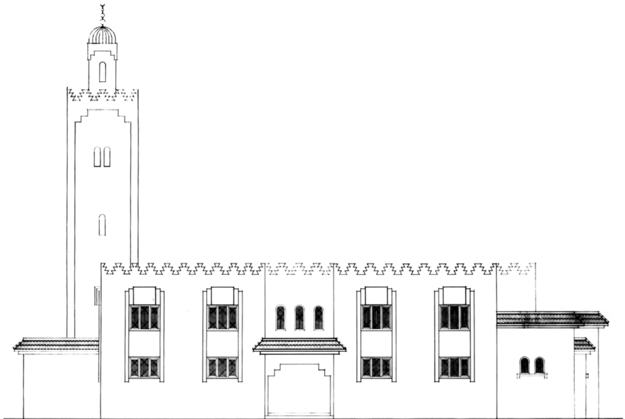
FACADE LATÉRALE GAUCHE
