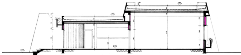
COUPE BB
