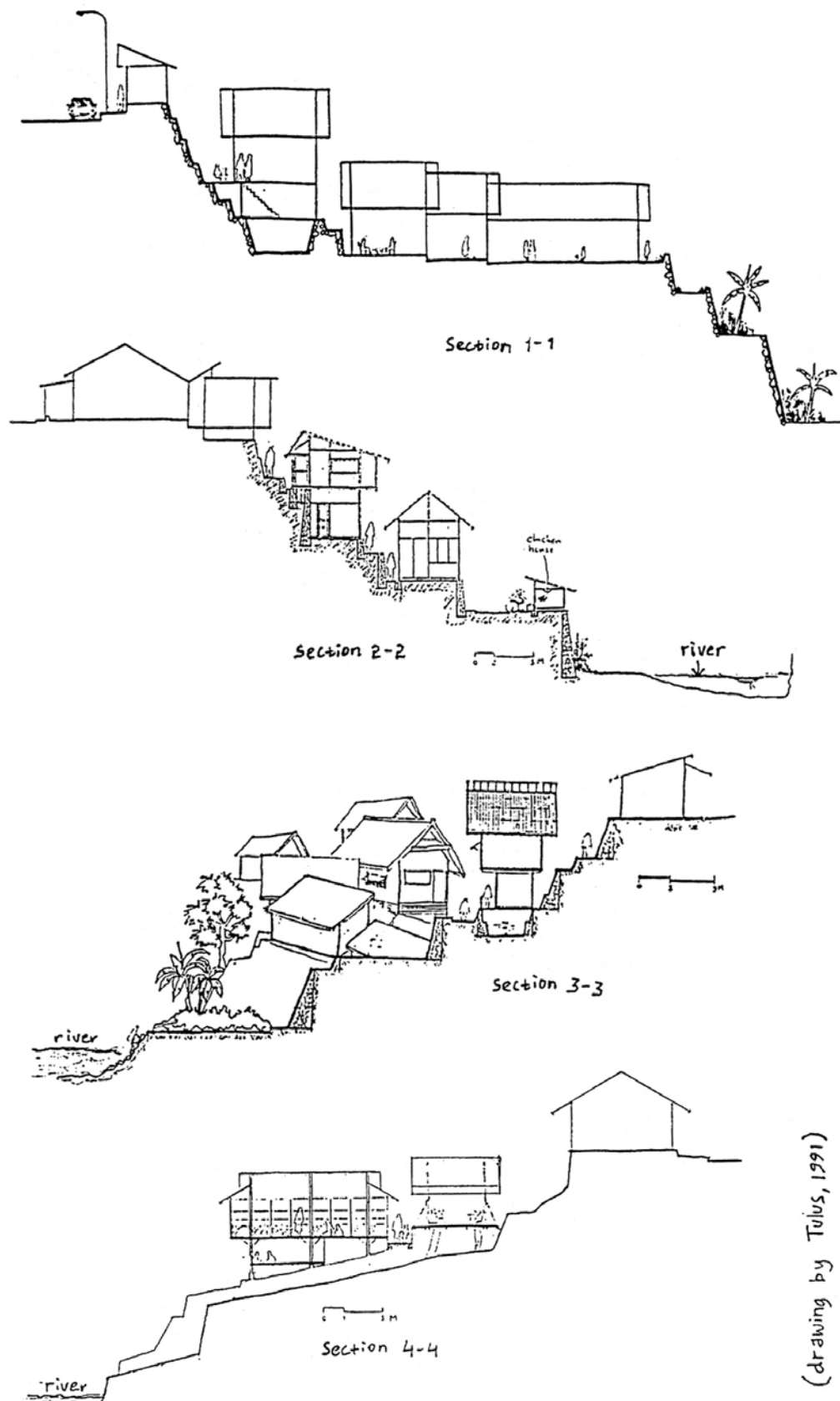
Fig. 4 : Site Section
