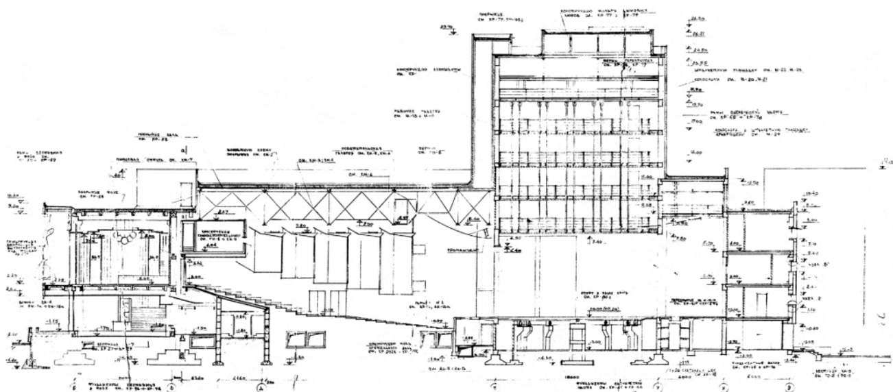
Section I - I 1:200
