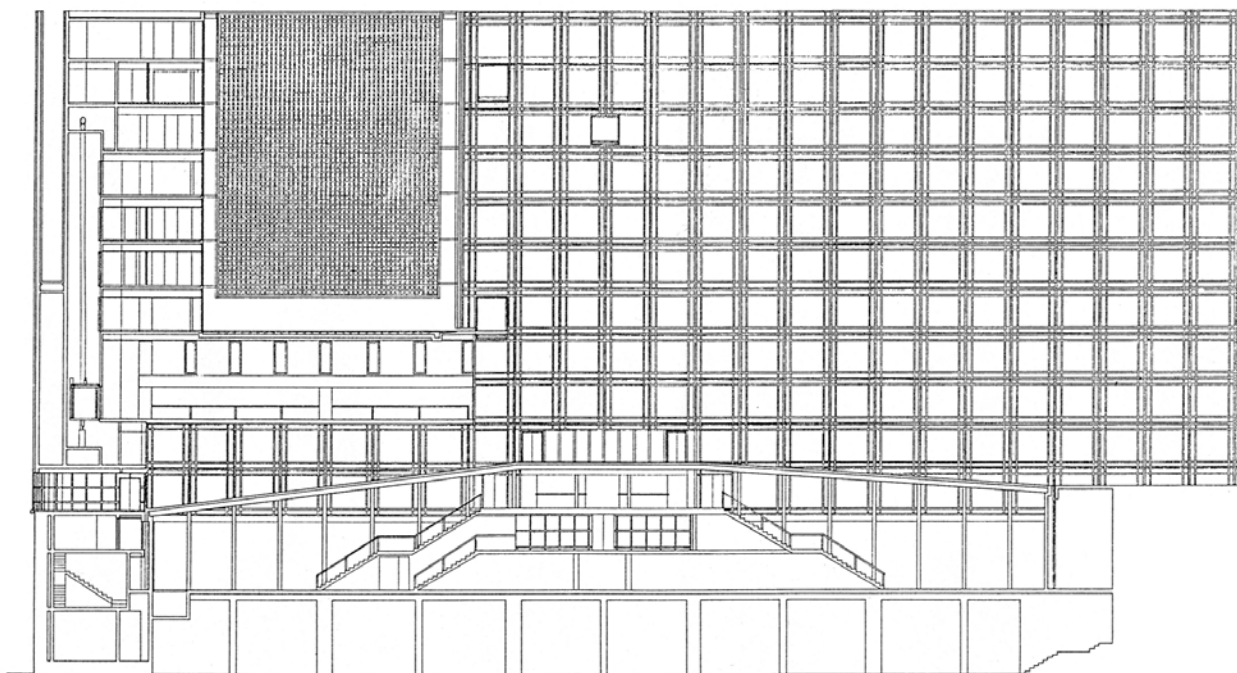
COUPE LONGITUDINALE SUR FAILLE
