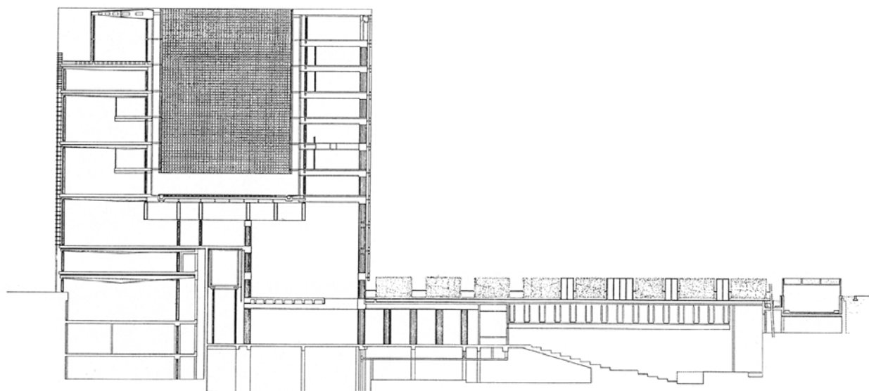
COUPE TRANSVERSALE SUR PATIO ET AUDITORIUM
