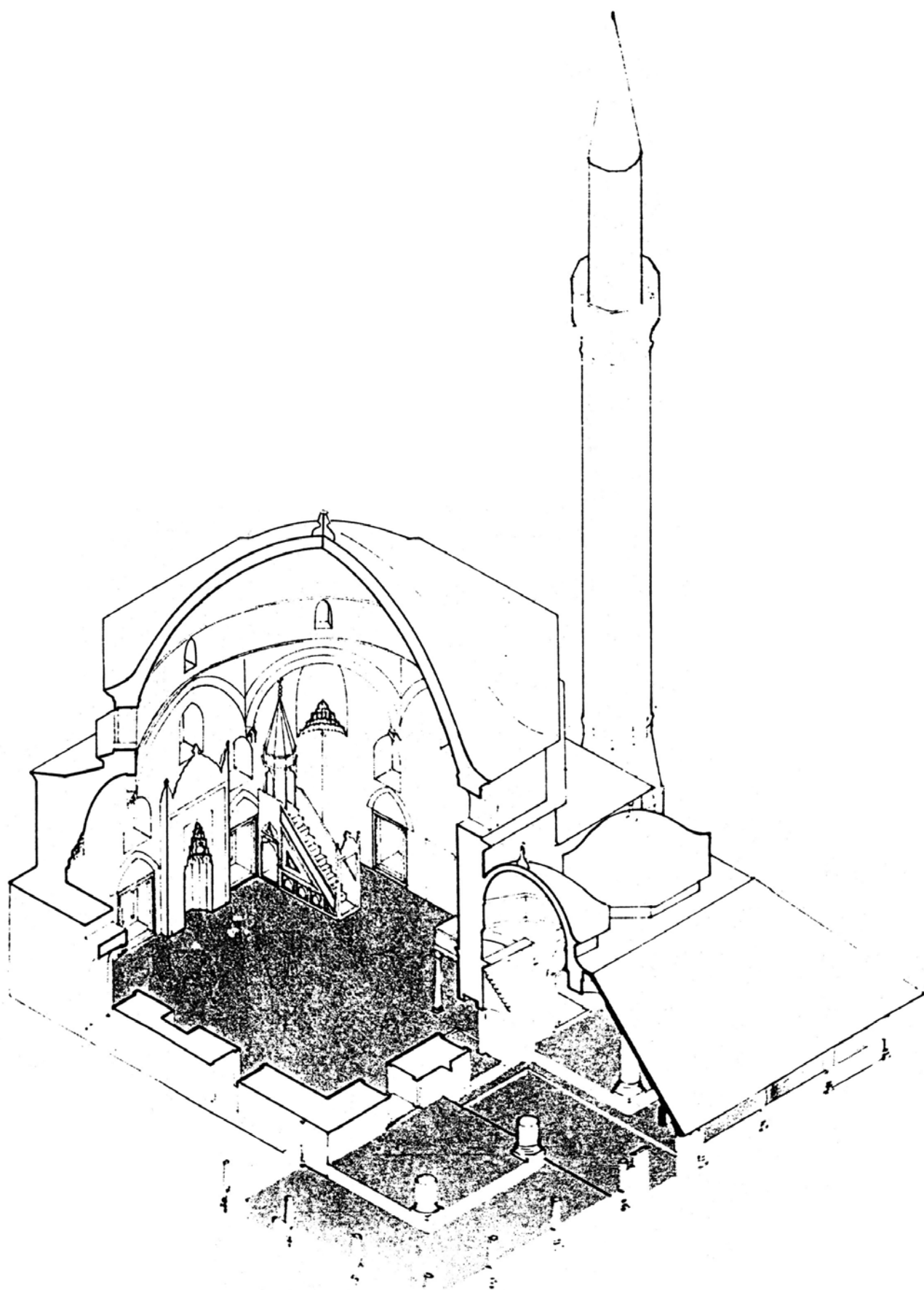
KARADŽOZBEGOVA DŽAMIJ IZOMETRIJSKI PRESJEK
