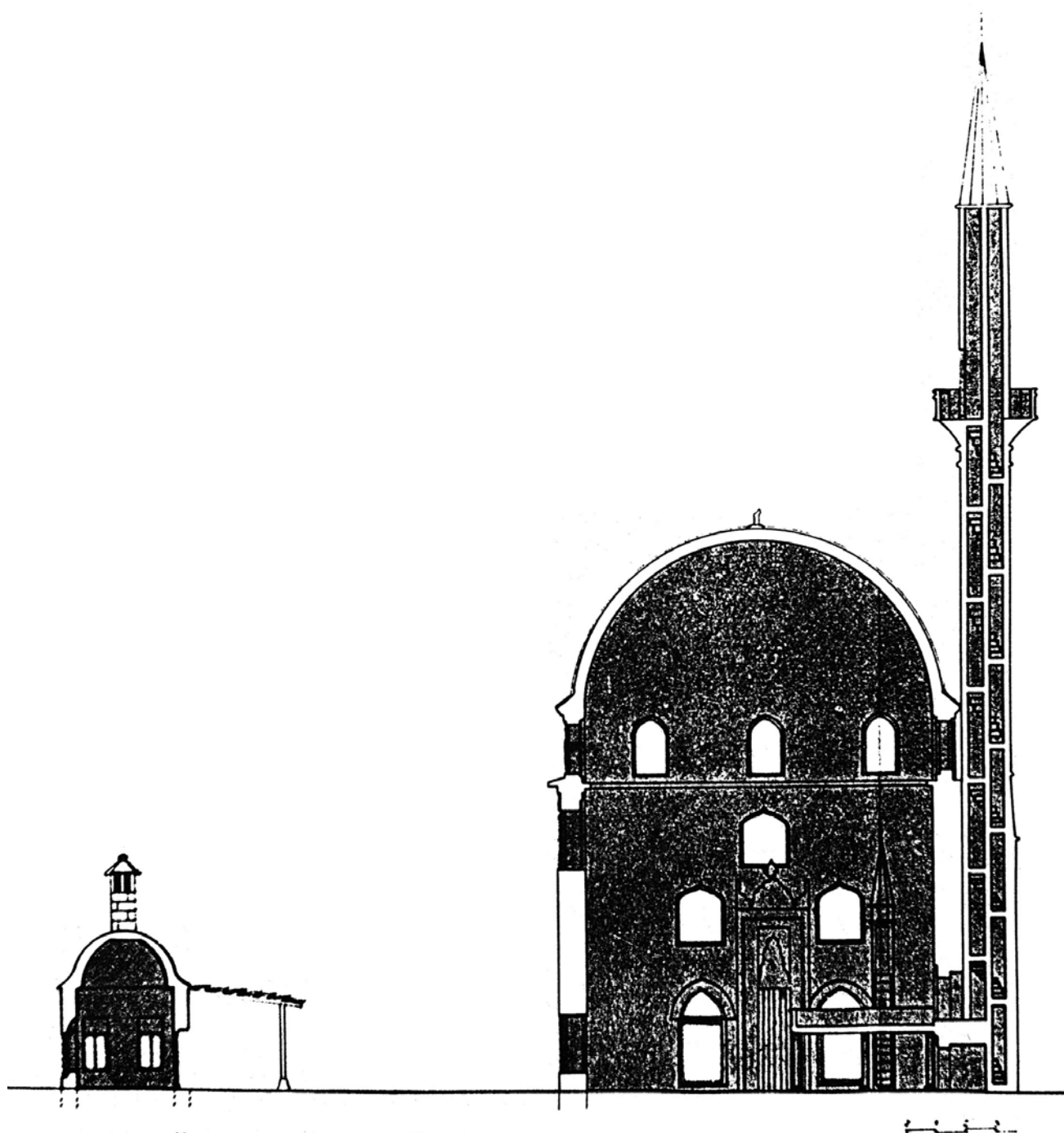
KARADŽOZBEGOVA DŽAMIJA I MEDRESA PRESJECI
