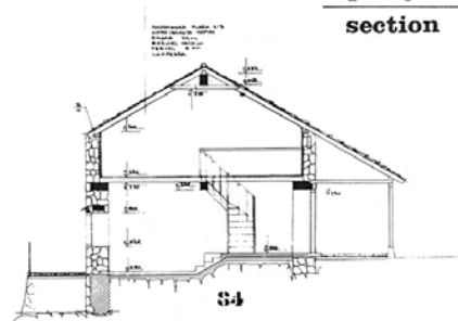
presjek section 84
