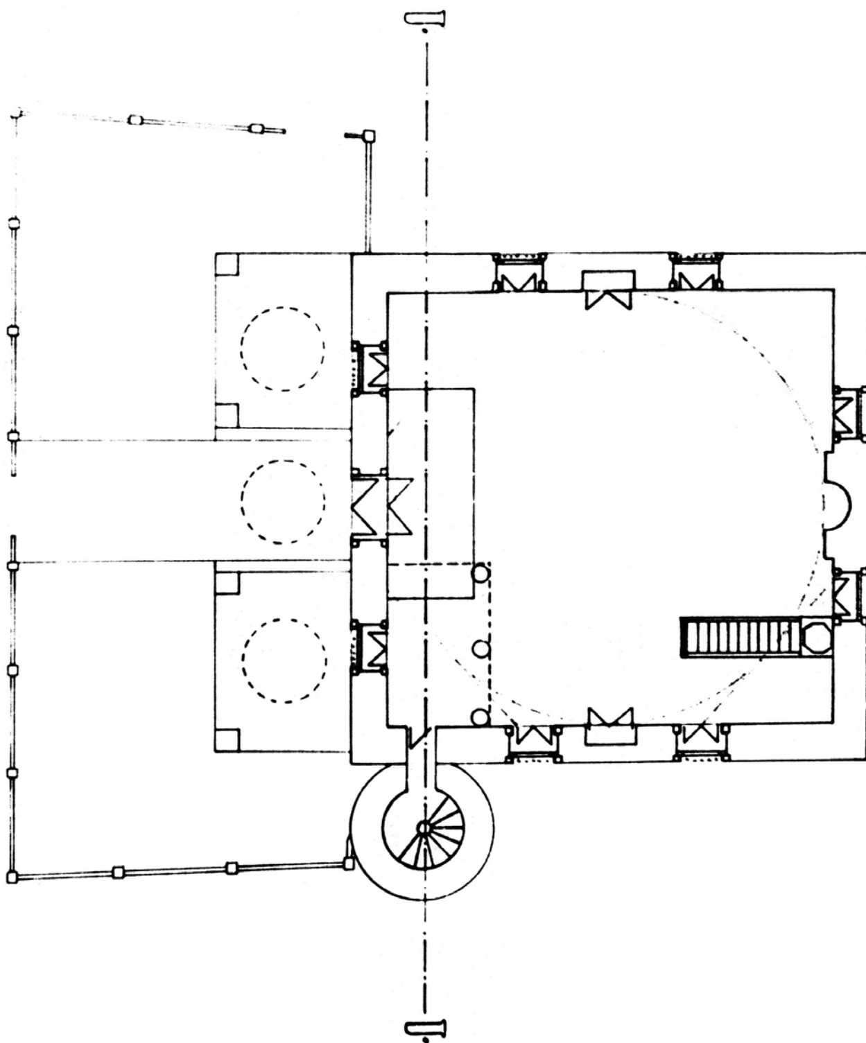
KARADŽIĆ-OZBEŽEVA DŽAMIJA OSNOVA
