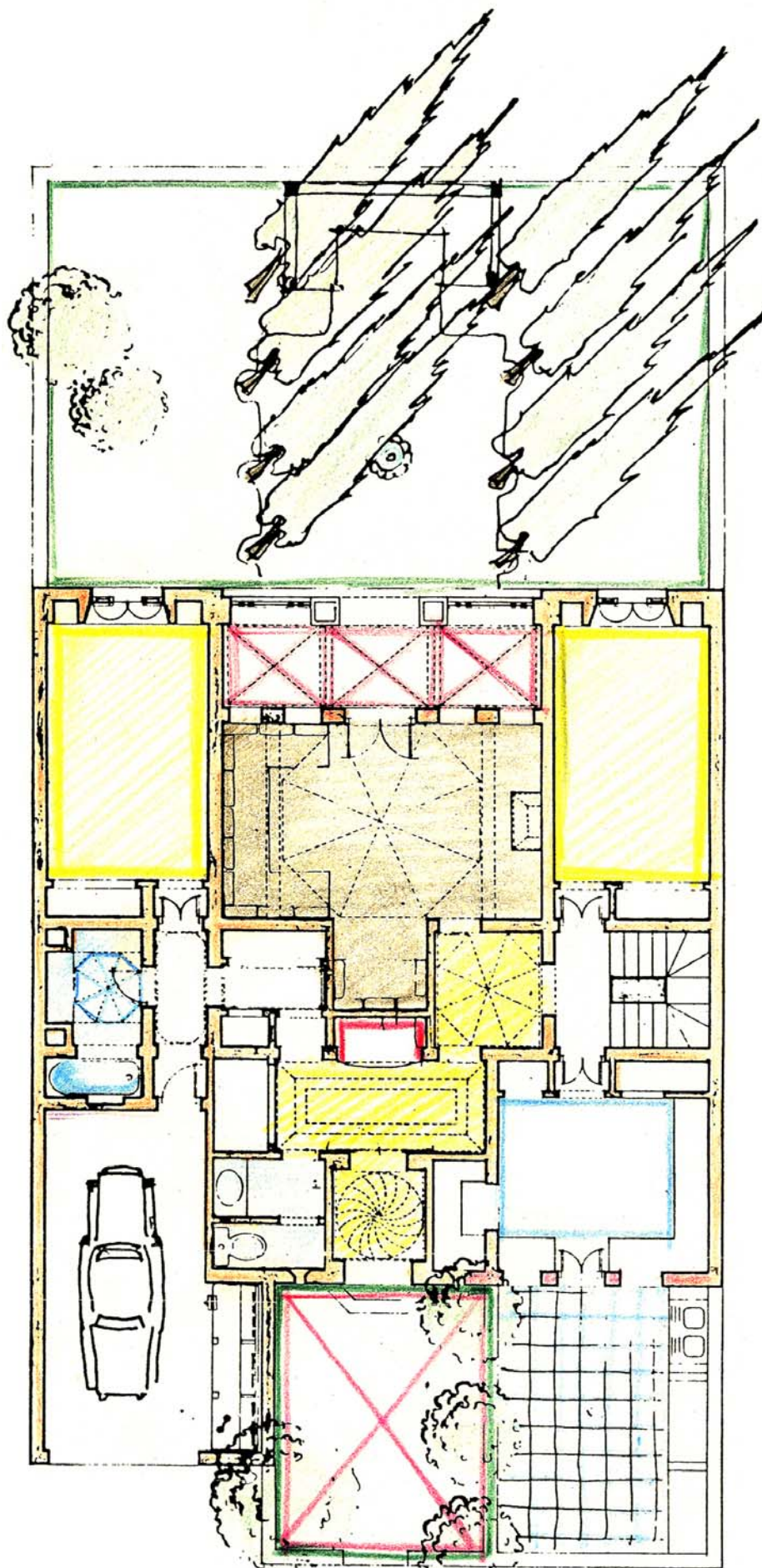
Maison en bande: rez-de-chaussée
