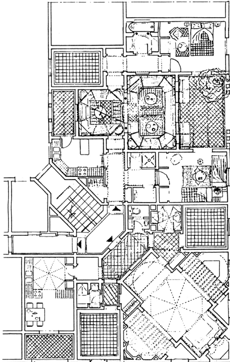
Assif Collectif : Deux appartements types
