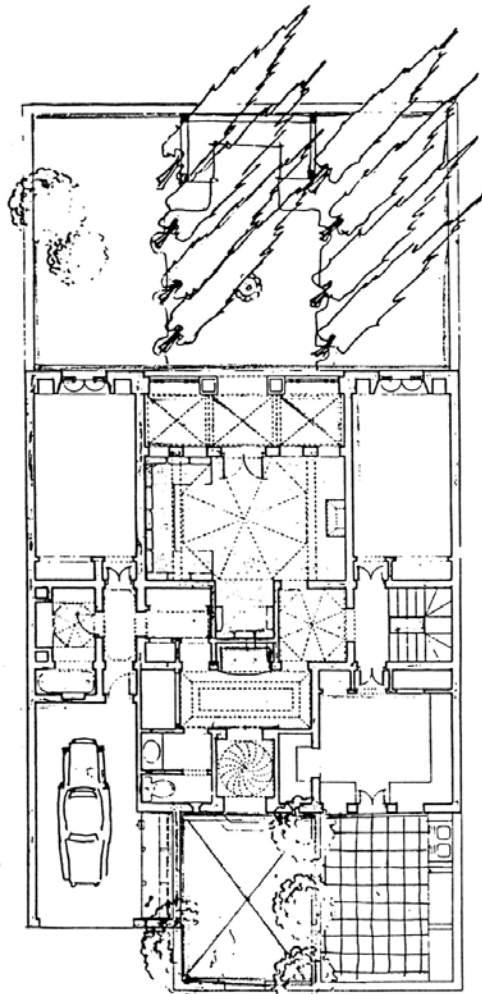
Maison en bande : Rez-de-chaussée
