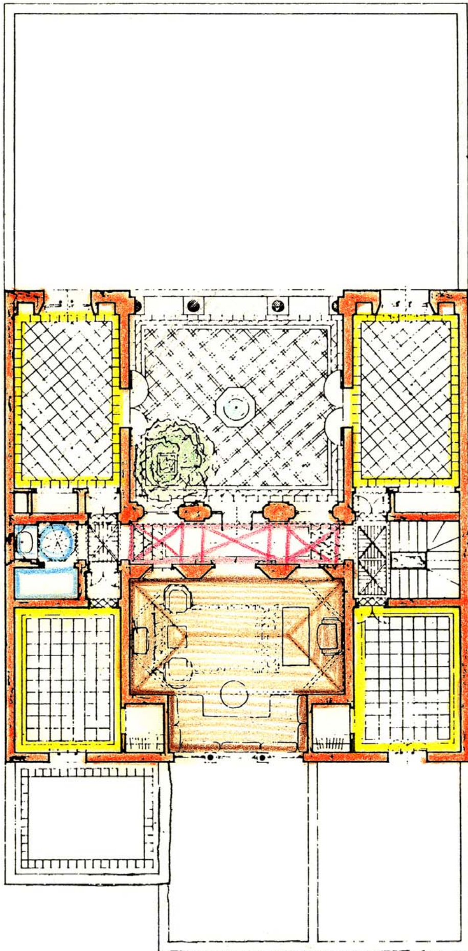
Maison en bande: étages avec patio haut
