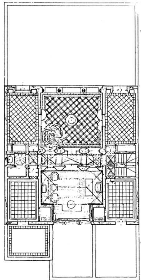
Maison en bande : Etage avec patio haut
