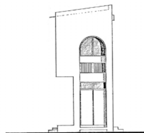
Elevation côté Nord
