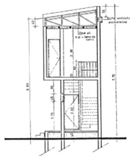
Coupe A-A
