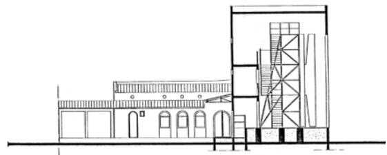
COUPE D-D
