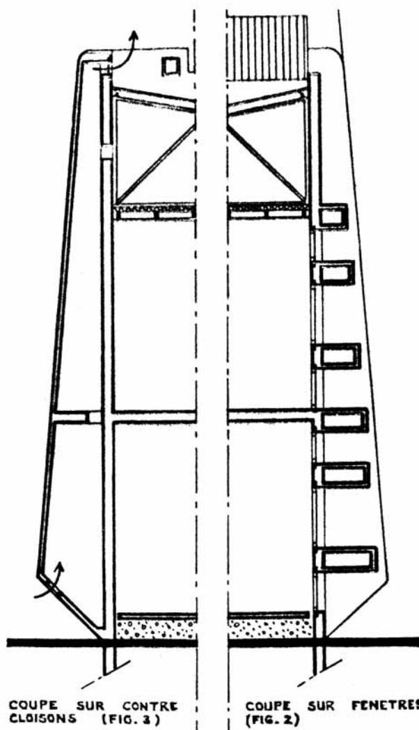
DETAILS LOGEMENS CHERCHEURS
