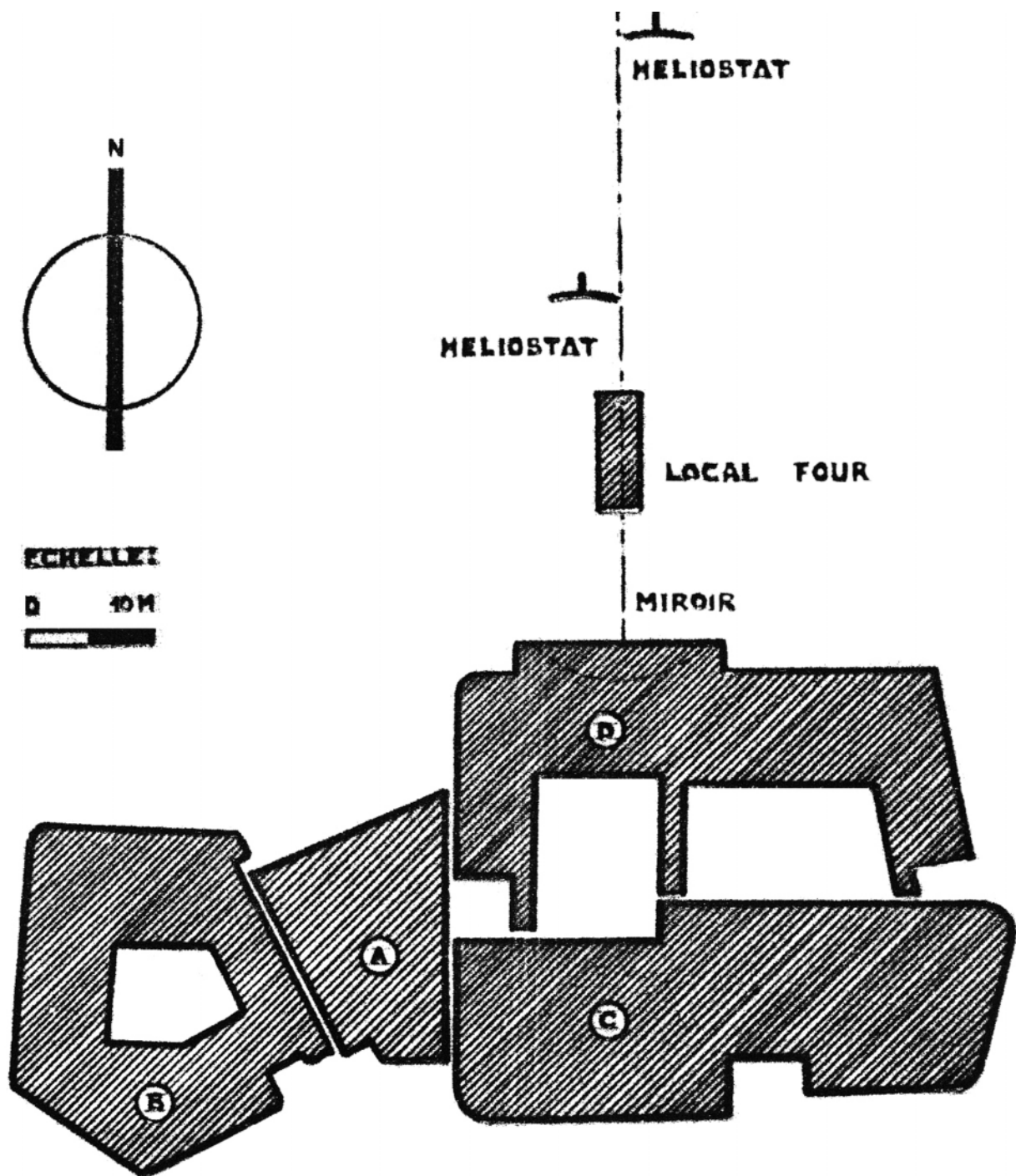
PLAN DE MASSE (FIG. 1)
