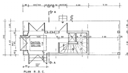
PLAN R.D.C.
