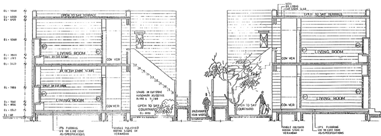
LONGITUDINAL SECTION A2 TYPE UNIT Scale 1:50
