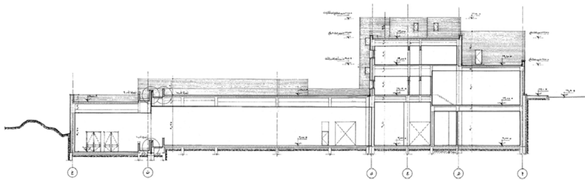
قطاع ب - ب
