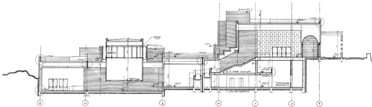
قطاع ٢ - ٢
