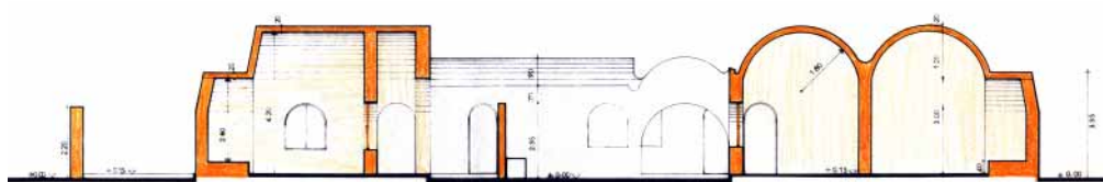
COUPE a-a 1:50
