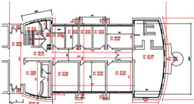
Rez-de-chaussée
