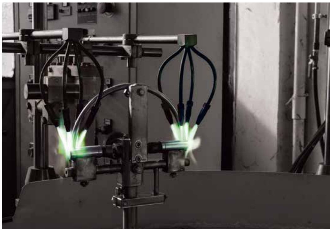
Ribrucciatura e sagomatura bordo vetro Gradi / Gradi glass rim glazing and shaping / Neubrennen und Formung des Glas-Rands der Gradi / Rebrûlage et moulure du bord du verre Gradi / Pulido al fuego y perfilado borde vidrio Gradi Saldobrasatura automatica archetto Gradi / Automatic Gradi arc brazing / Automatisches Hartlöten des Bogens der Gradi / Soudo-brasage automatique du petit arc Gradi / Soldadura automática fuerte por aleación arco Gradi
