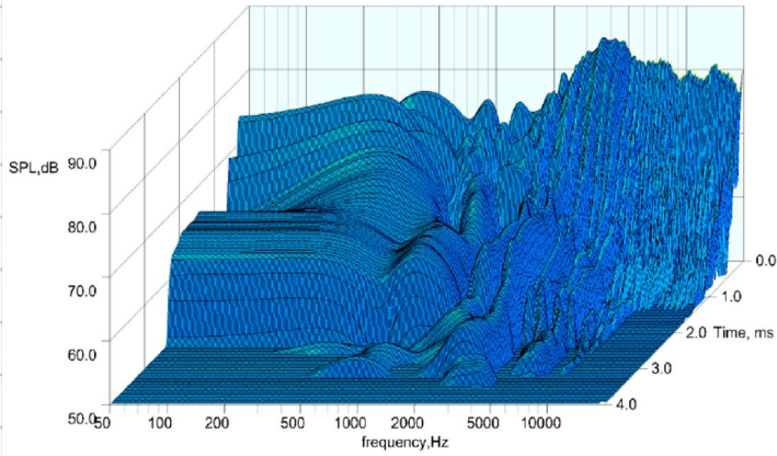
Waterfall Graph 70 Volt
