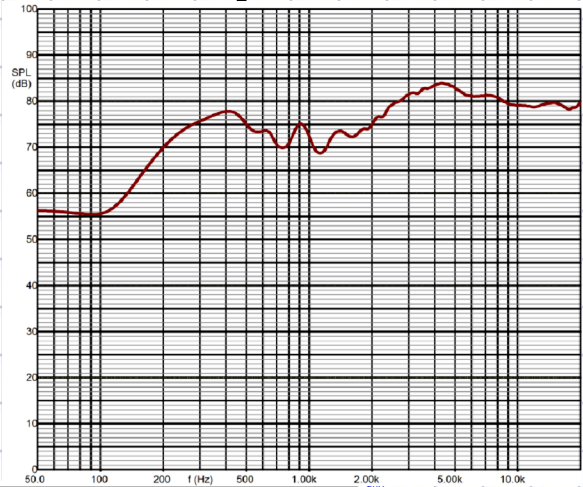
SPL-Response 70 Volt
