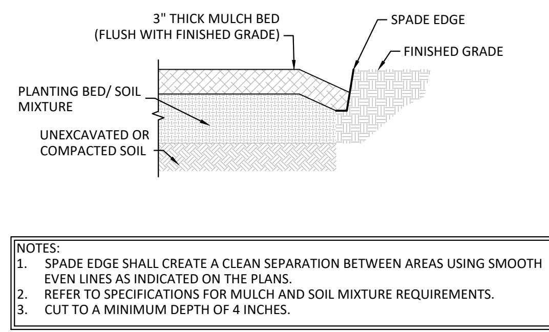
5 SPADE EDGE DETAIL NO SCALE
