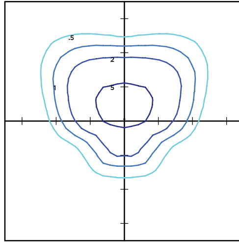
ISO FOOTCANDLE
