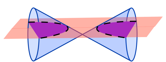
Hyperbola
