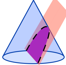
Parabola
