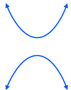
Hyperbola
