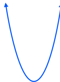
Parabola
