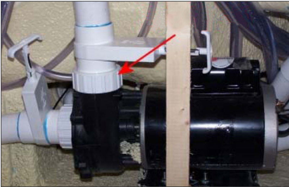
FIGURE 1.5 : BAGUE DE POMPE; DESERRERZ POUR LAISSER S'ÉCHAPPER L'AIR
