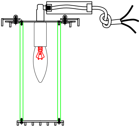
03-Lamp Body
