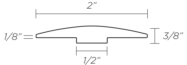
3/8" T-Mold - 78" long
