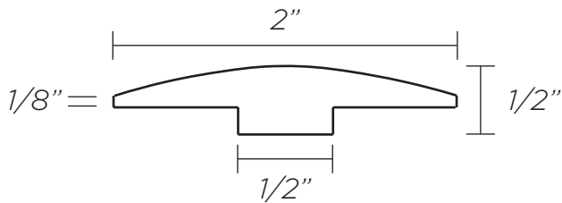
1/2" T-Mold - 78" long
