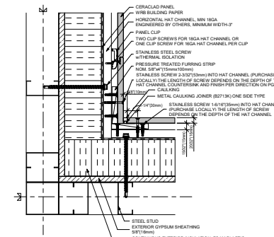
5 INSIDE CORNER (STEEL STUD)
