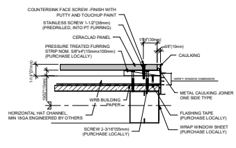
8 WINDOW AND DOOR JAMB (STEEL STUD)
