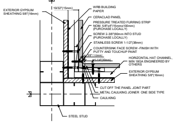
5 INSIDE CORNER (STEEL STUD)
