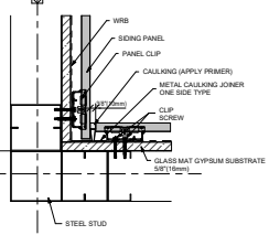
5 INSIDE CORNER (STEEL STUD)
