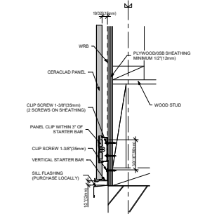
1 STARTER BAR (STEEL STUD)
