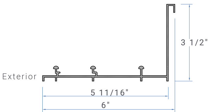
Frame sill standard sliding door
