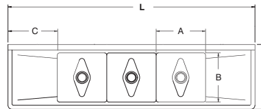
3 COMP - 2 DRBD
