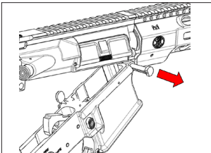
Pull pivot pin.
