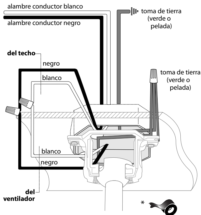
(cableado para el ventilador)
