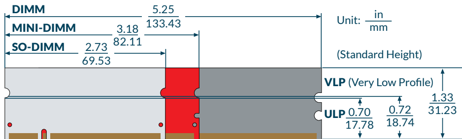
DDR4 JEDEC MODULE DIMENSIONS
