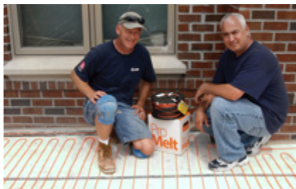
ProMelt ® Cable
