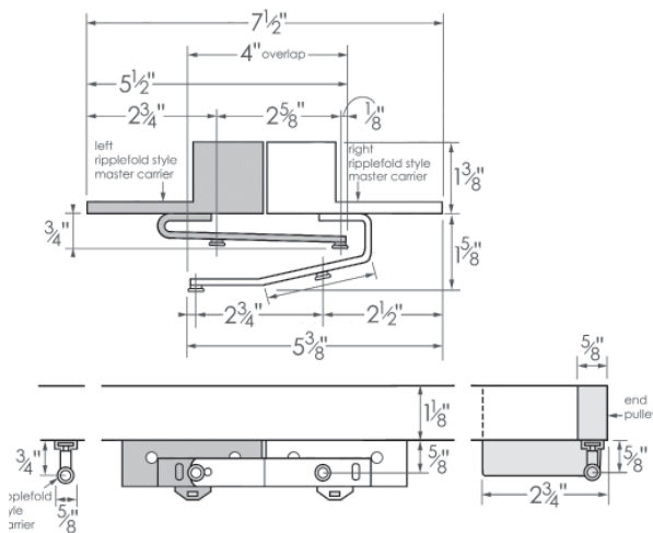
Ripplefold® style
